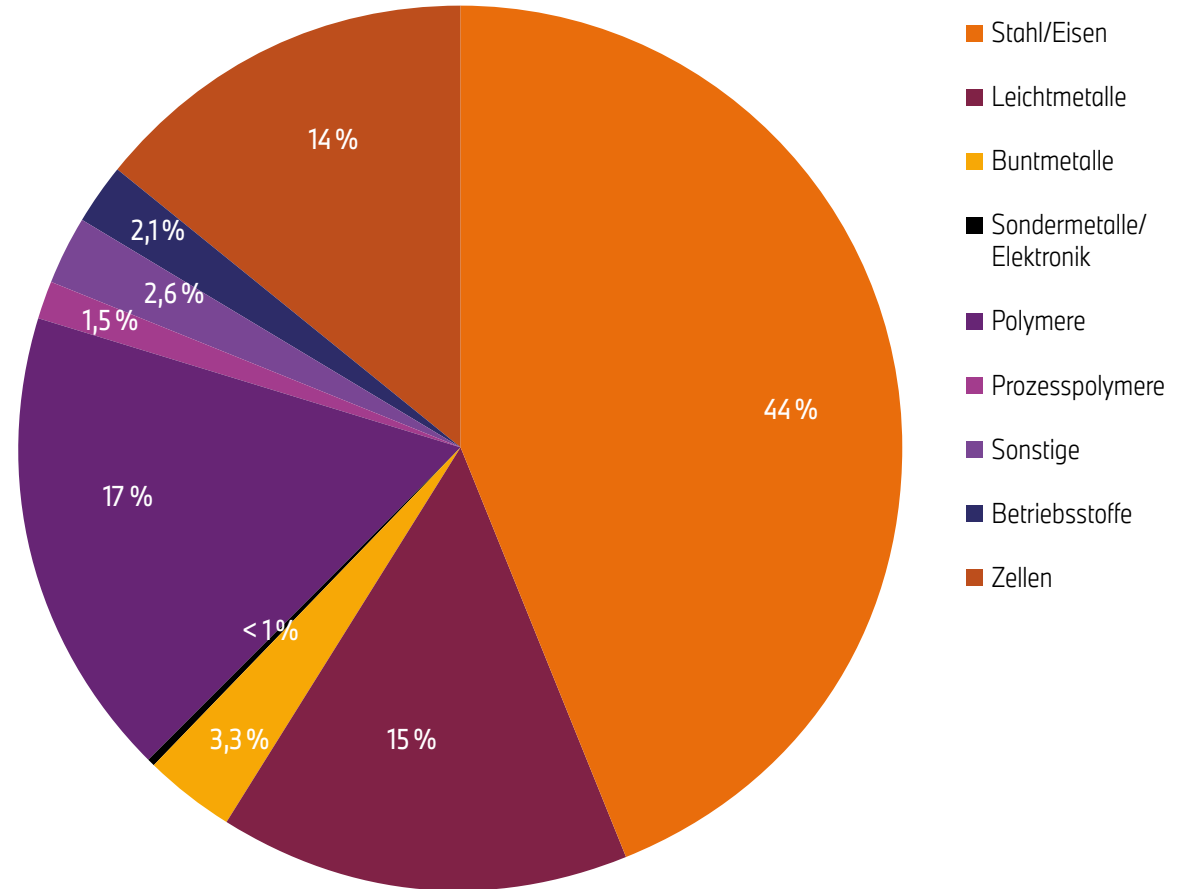
Abb. 2: Werkstoffzusammensetzung des Countryman E zum Produktionsstart. Die angegebenen Werte können Rundungsdifferenzen aufweisen.
