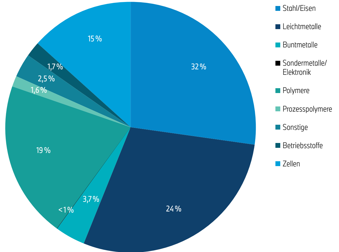
Abb. 2: Werkstoffzusammensetzung des BMW i5 eDrive40 zum Produktionsstart. Die angegebenen Werte können Rundungsdifferenzen aufweisen.
