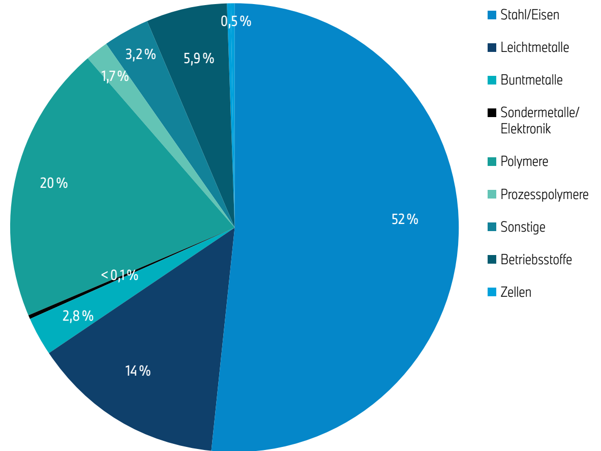
Abb. 2: Werkstoffzusammensetzung des BMW X3 20d xDrive zum Produktionsstart. Die angegebenen Werte können Rundungsdifferenzen aufweisen.
