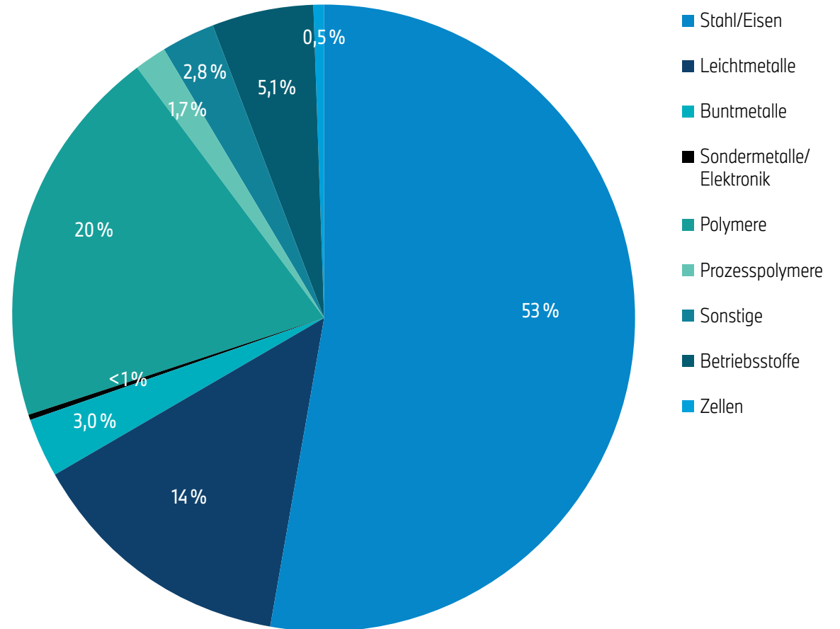
Abb. 2: Werkstoffzusammensetzung des BMW X3 20 xDrive zum Produktionsstart. Die angegebenen Werte können Rundungsdifferenzen aufweisen.
