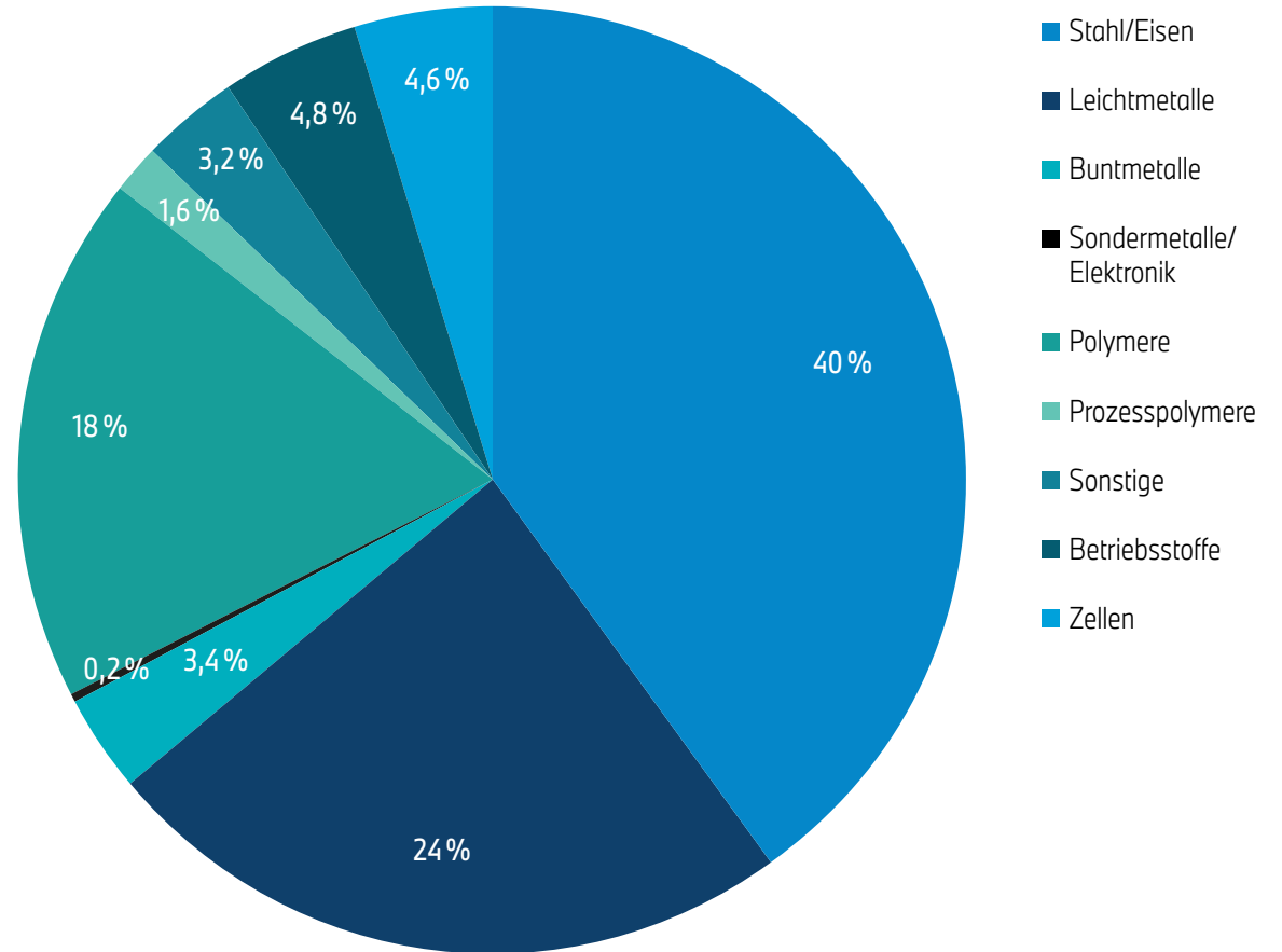
Abb. 2: Werkstoffzusammensetzung des BMW 530e zum Produktionsstart. Die angegebenen Werte können Rundungsdifferenzen aufweisen.
